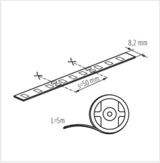
LEDS-B4,8W/M12IP65-NW
