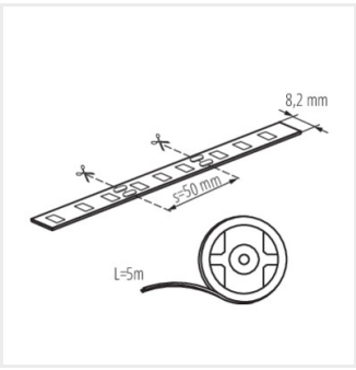
LEDS-B4,8W/M12IP65-CW
