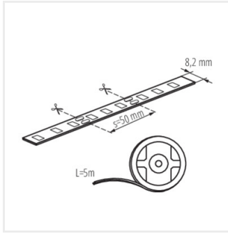
LEDS-B4,8W/M12IP65-WW
