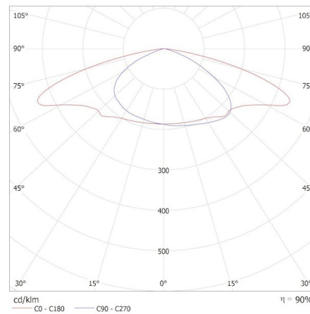
KANLUX S.A. (kat 39281) PRO-S M 75W NW / Krzywa rozsytu światła (biegunowo)
