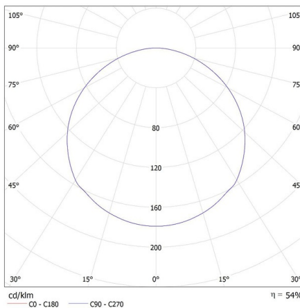
KANLUX S.A. (kat 38931) ANBAR LED 37W CCT W 4000K / Krzywa rozsytu światła (biegunowo)
