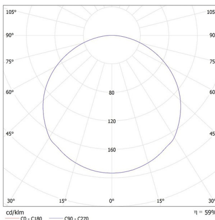
KANLUX S.A. (kat 38931) ANBAR LED 37W CCT W 4000K / Krzywa rozsytu światła (biegunowo)
