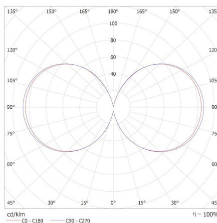
KANLUX S.A. (kat 37349) XLED HP EX E40 43W-NW / Krzywa rozsyłu światła (biegunowo)
