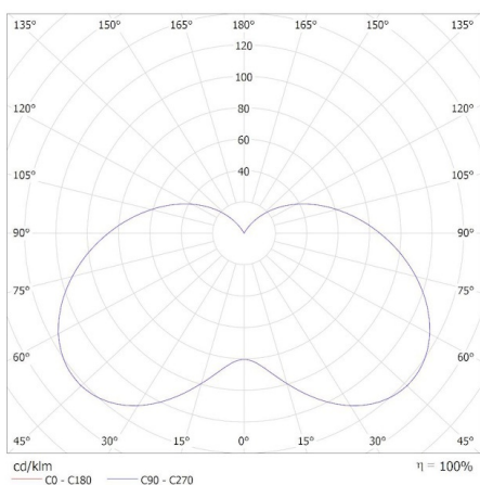
KANLUX S.A. (kat 36682) IQ-LED C35E14 3,4W-WW / Krzywa rozsytu światła (biegunowo)
