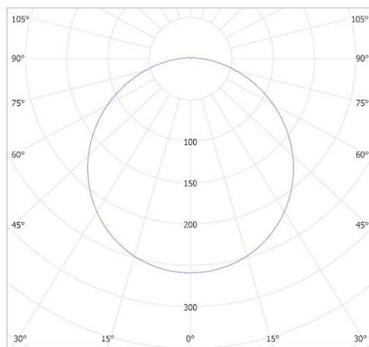
KANLUX S.A. (kat 35005) STIVI LED 10W-NW-O-SE / Krzywa rozsyłu światła (biegunowo)
