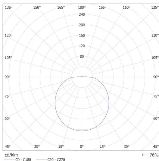
KANLUX S.A. (kat 26785) AVAR O 6060 40W-NW / Krzywa rozsyłu światła (biegunowo)
