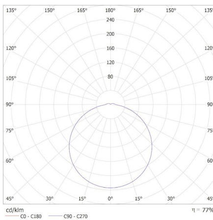
KANLUX S.A. (kat 37297) IPER LED 35W-NW-L / Krzywa rozsyłu światła (biegunowo)
