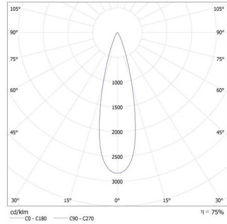
KANLUX S.A. (kat 35653) BTL 18W-940-B 15deg + GRID / LDC (Polar)
