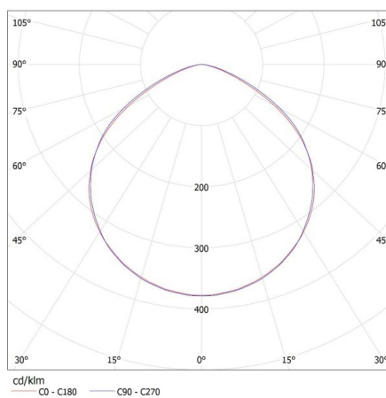
KANLUX S.A. (kat 33204) ANTEM LED 100W-NW B / LDC (Polar)
