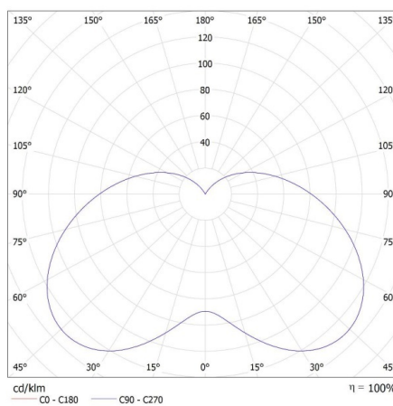
MILED0 (kat 31307) C35 N 4,9W E14-WW / LDC (Polar)
