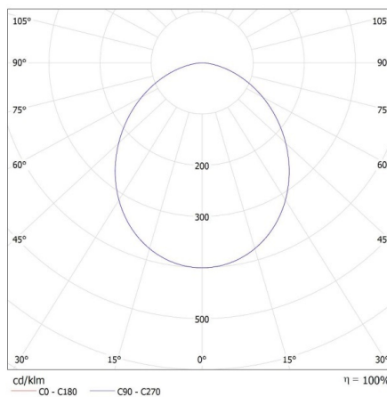
MILEDO (kat 31236) GU10 8W-WW LED / LDC (Polar)
