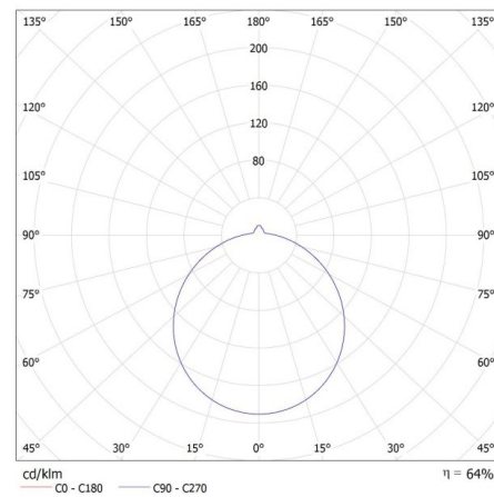
MILED0 (kat 31222) CORSO LED V2 24-NW / LDC (Polar)
