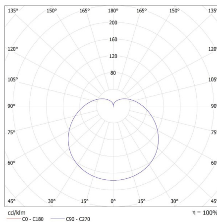
MILED0 (kat 31207) A60 N 13W E27-NW / LDC (Polar)
