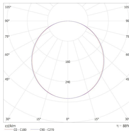
MILED0 (kat 31174) BAREV BL 40W 12030 NW / Krzywa rozsytu światła (biegunowo)
