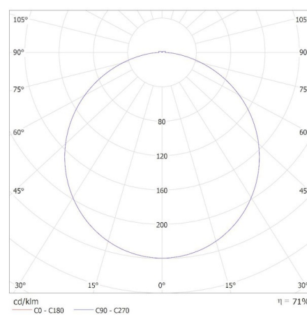
KANLUX S.A. (kat 26777) AVAR 6262 28-40W-NW / Krzywa rozsyłu światła (biegunowo)
