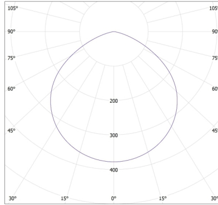
KANLUX S.A. (kat 15098) RANGO R7S SMD-WW / Krzywa rozsyłu światła (biegunowo)
