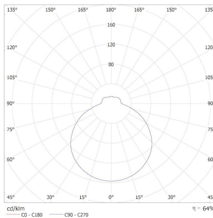
KANLUX S.A. (kat 37320) LUMKO LED 17,5W NW / Krzywa rozsytu światła (biegunowo)
