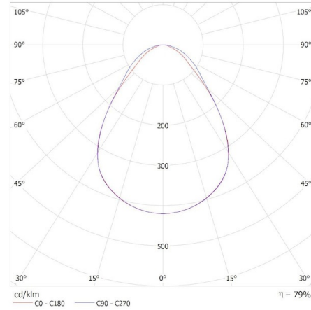
KANLUX S.A. (kat 37179) BLINGO U24W 4000 60NW / Krzywa rozsytu światła (biegunowo)
