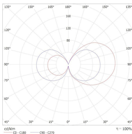
KANLUX S.A. (kat 36243) XLED EX A60 4W-WW / Krzywa rozsytu światła (biegunowo)
