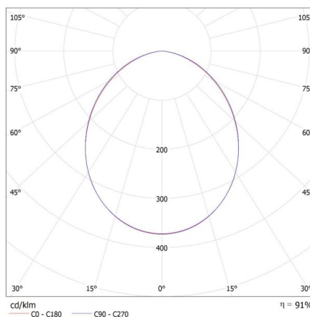
KANLUX S.A. (kat 33883) IQ-LED FL-50W-NW / LDC (Polar)
