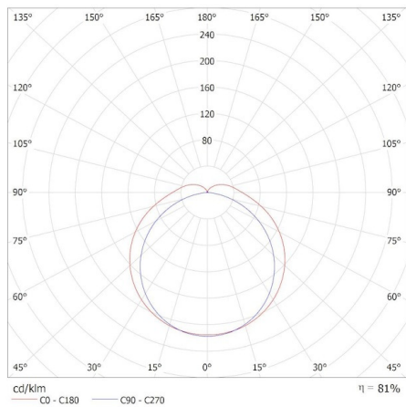
KANLUX S.A. (kat 33173) TP STRONG ECO 46W-NW / Krzywa rozsytu światła (biegunowo)
