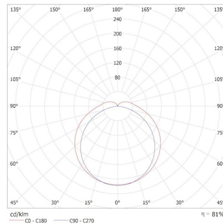
KANLUX S.A. (kat 33173) TP STRONG ECO 46W-NW / Krzywa rozsyłu światła (biegunowo)
