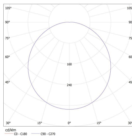
KANLUX S.A. (kat 32530) DROMI LED EL-1 7W-GR / LDC (Polar)
