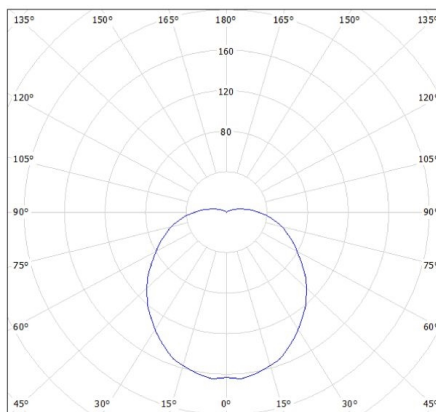
KANLUX S.A. (kat 18120) FOGLER DL-2400 / Krzywa rozsyłu światła (biegunowo)
